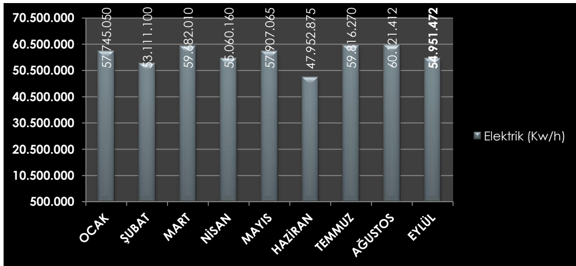
Grafik 12 – 2017 Konya Organize Sanayi Bölgesi Elektrik Tüketim Verileri (Kw/h)
